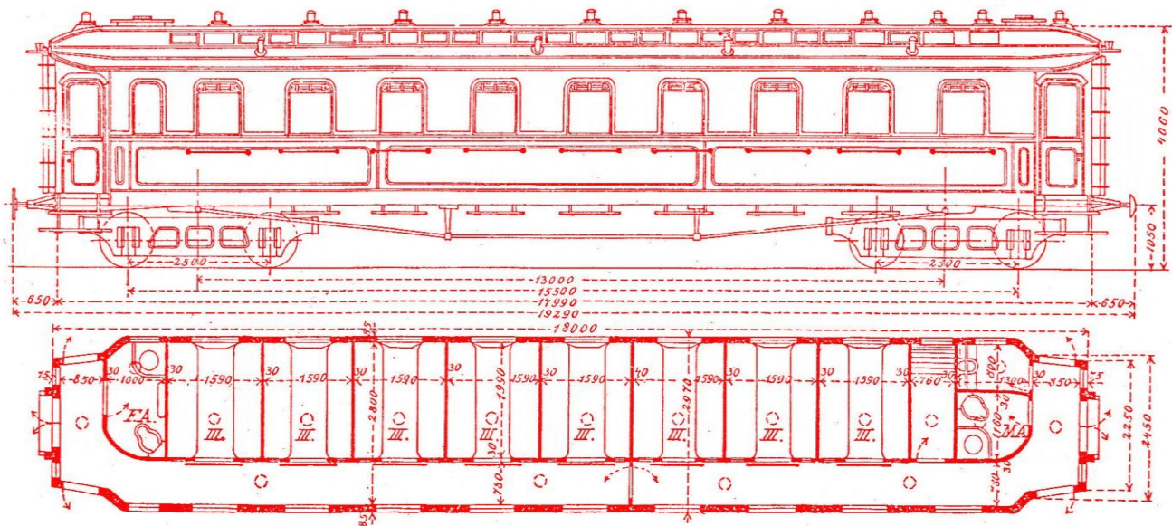
Skizze 177 C 4ü der Gattung S 2 nach Musterblatt D I 6 und Ia 6, gebaut 1902–1908
