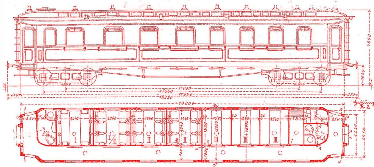
Skizze 176 ABC 4ü der Gattung R 2 nach Musterblatt I a 5, gebaut 1903–1904
