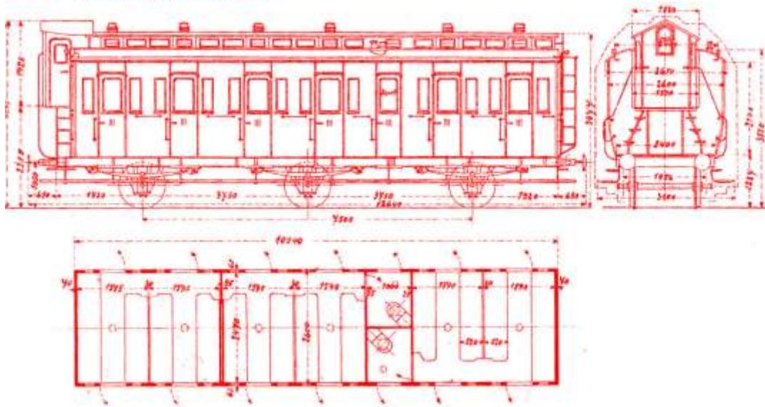
Skizze 99 C3 nach Blatt Ib 9a von 1908
