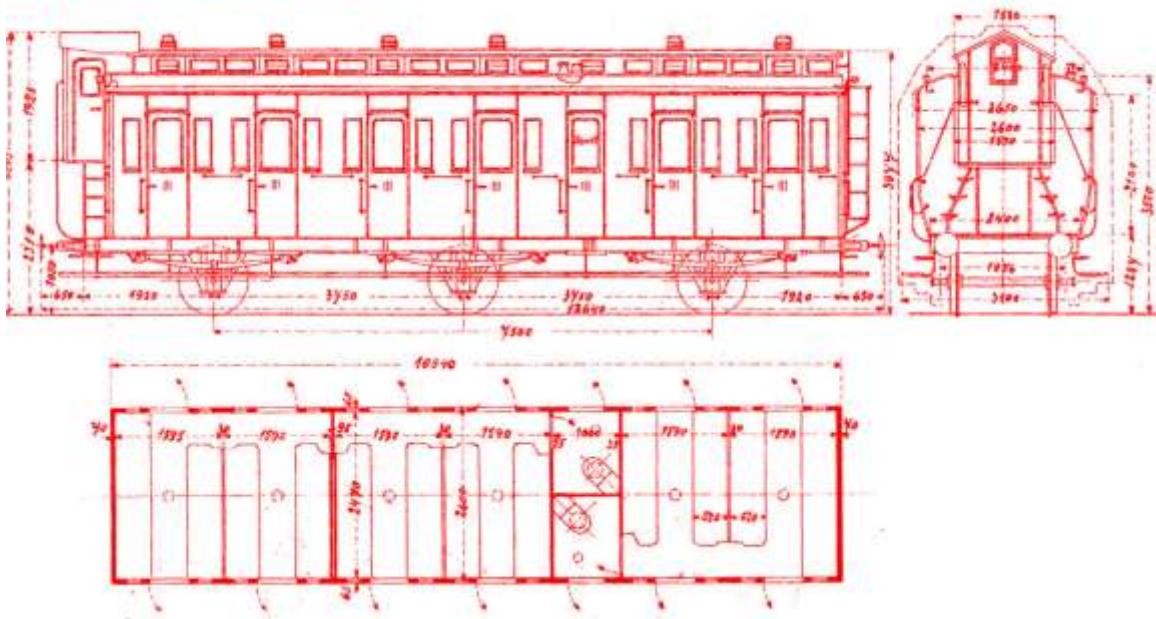
Skizze 99 C3 nach Blatt Ib 9a von 1908
