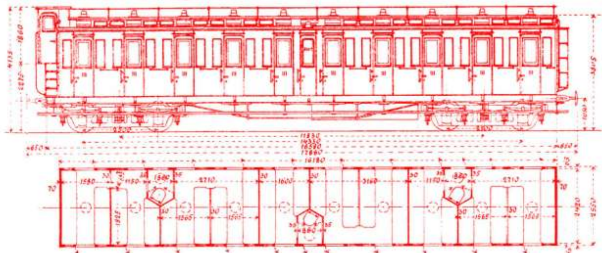
Skizze 117 C4 nach Blatt 3093 B, gebaut ab 1896
