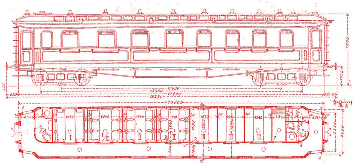
Skizze 176 ABC 4 ü der Gattung R 2 nach Musterblatt I a 5, gebaut 1903-1904
