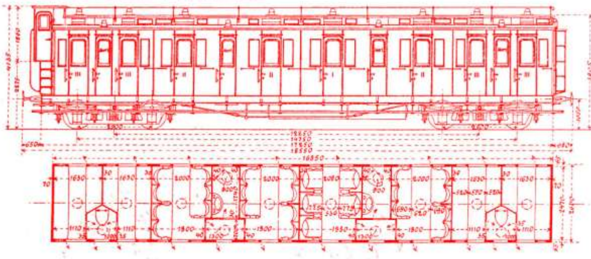
Skizze 119 ABC 4 nach Blatt DI 22, gebaut ab 1901
