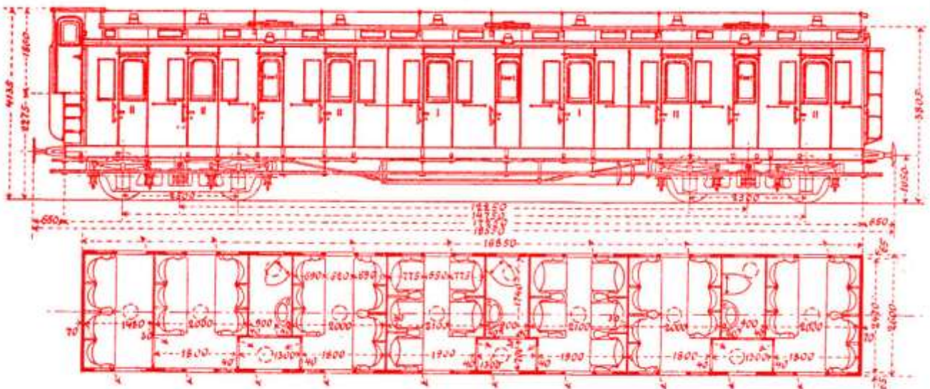
Skizze 118 AB4 nach Blatt DI 21, gebaut ab 1900
