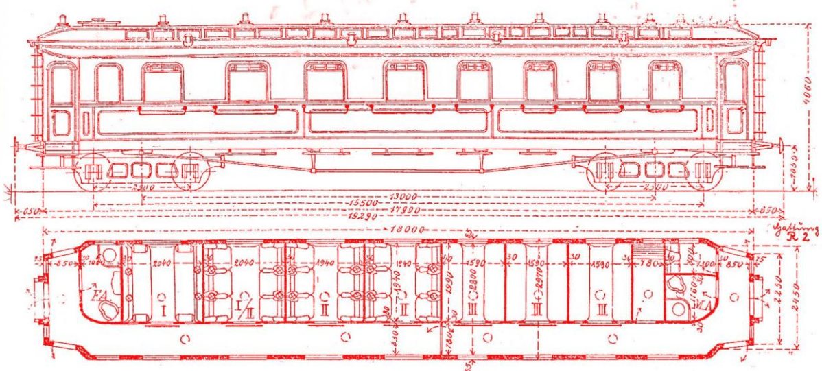
Skizze 176 ABC4u der Gattung R 2 nach Musterblatt I a 5, gebaut 1903–1904
