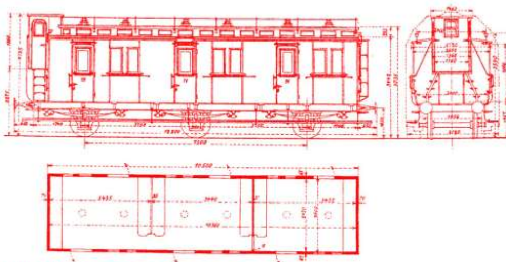
Skizze 90 D3 nach Blatt Bh 3 von 1900 (ohne Abort)
