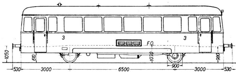
L ü b e c k - B ü c h e n e r - E i s e n b a h n Dieseltriebwagen VT 12
