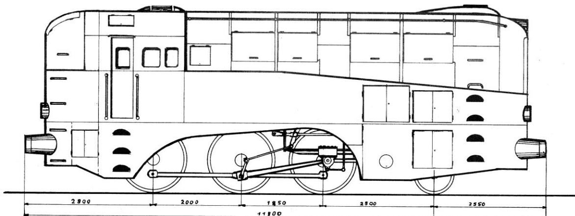
L ü b e c k - B ü c h e n e r - E i s e n b a h n 1 C Tenderlok, Gattung T 12, Stromlinie, Umbau von Lok 138 bis 142, Maße der Skizze Loks Pt 34,16
