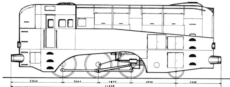
Lübeck - Büchener - Eisenbahn 1 C Tenderlok, Gattung T 12, Stromlinie, Umbau von Lok 138 bis 142, Maße der Skizze Loks Pt 34,16
